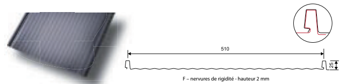
F - nervures de rigidité - hauteur 2 mm
