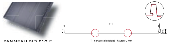
T - nervures de rigidité - hauteur 2 mm
